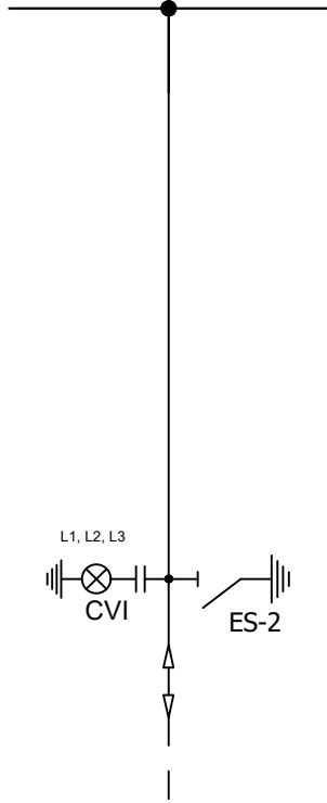
Tek Hat Şeması Single Line Diagram
