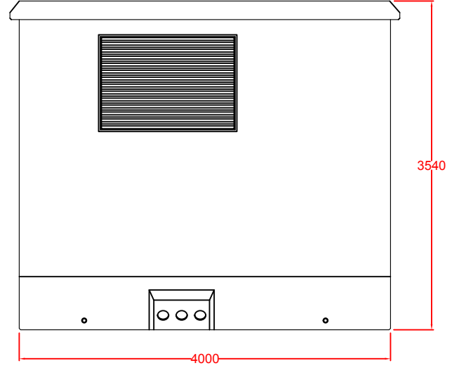
"B" GÖRÜNÜŞÜ "B" SECTION
