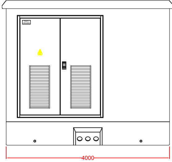
"A" GÖRÜNÜŞÜ "A" SECTION
