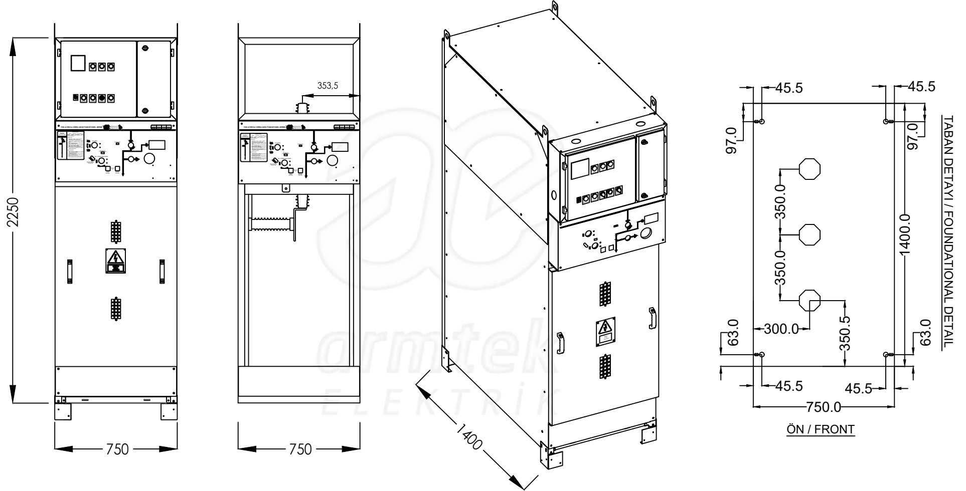
H01 : Hava Yalıtımlı Metal Mahfazalı Modüler Tip Yük Ayırıcılı Giriş-Çıkış Fonksiyonel Birimi (Air Insulated Metal Enclosed Modular Type Incoming-Outgoing Switchgear with Load Break Switch)
